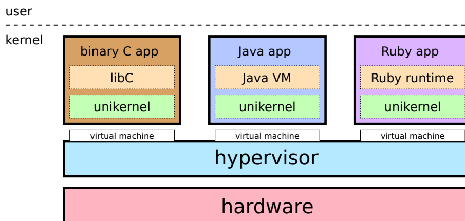
Figura 3.7: Sistema uninúcleo.
