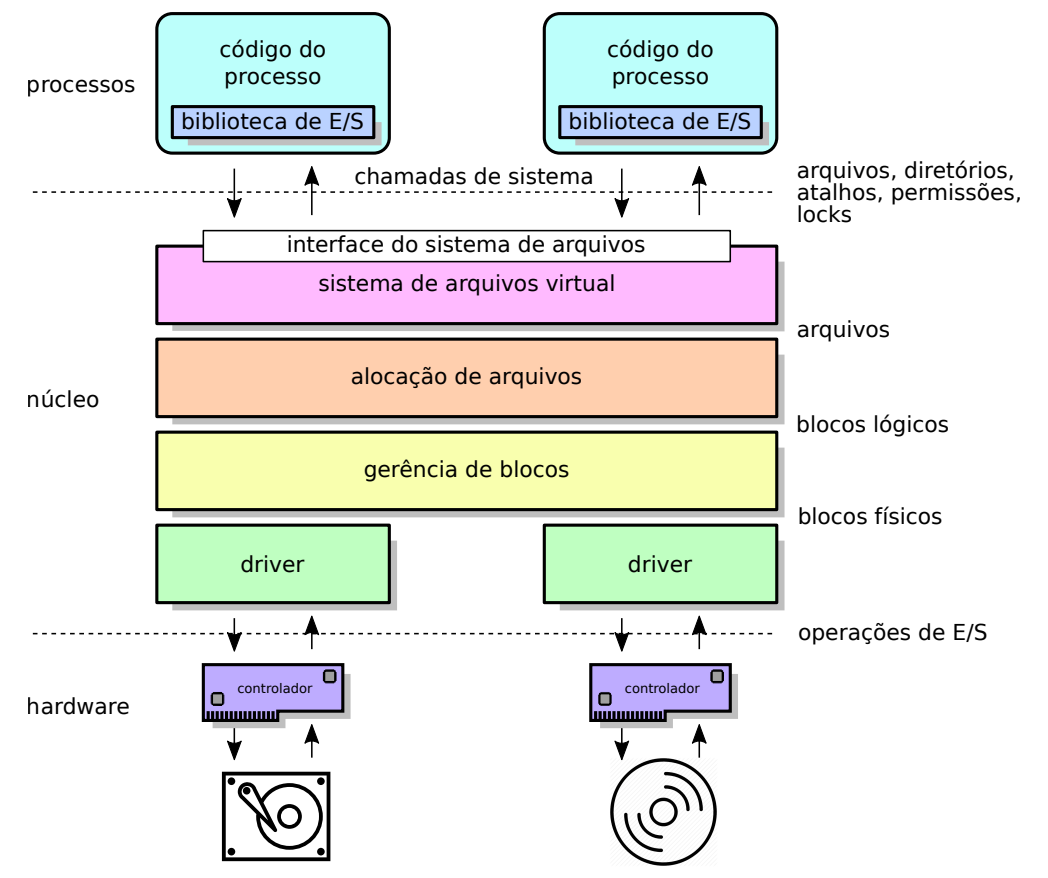
Figura 24.1: Camadas da implementação da gestão de arquivos.
