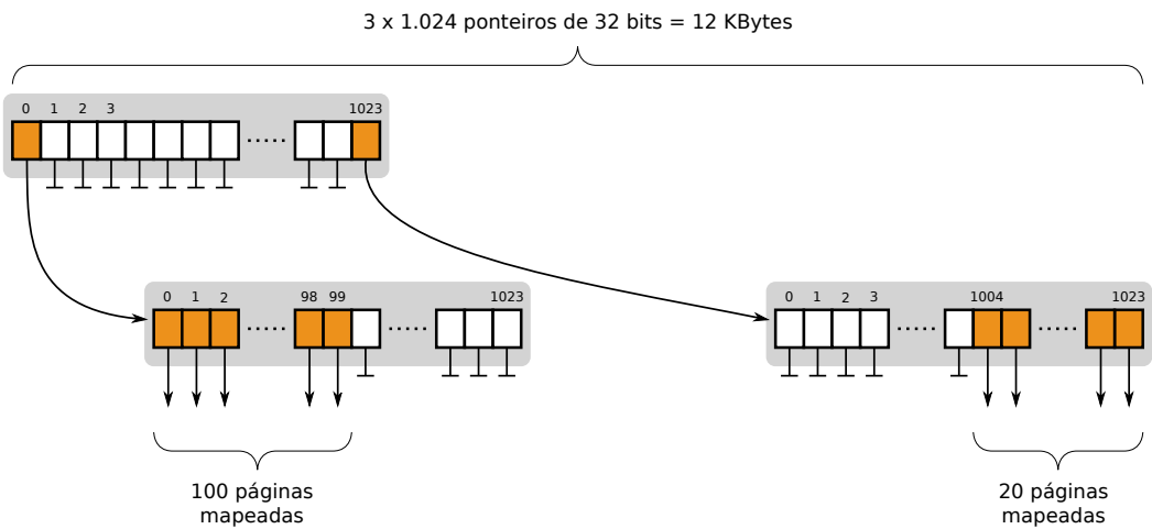
Figura 14.11: Tabela de páginas com dois níveis.
