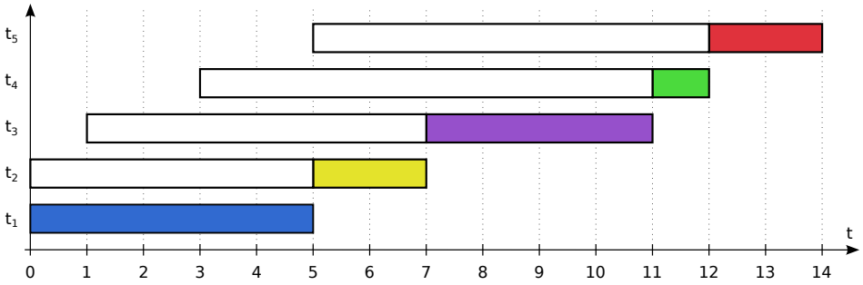
Figura 6.1: Escalonamento FCFS.
