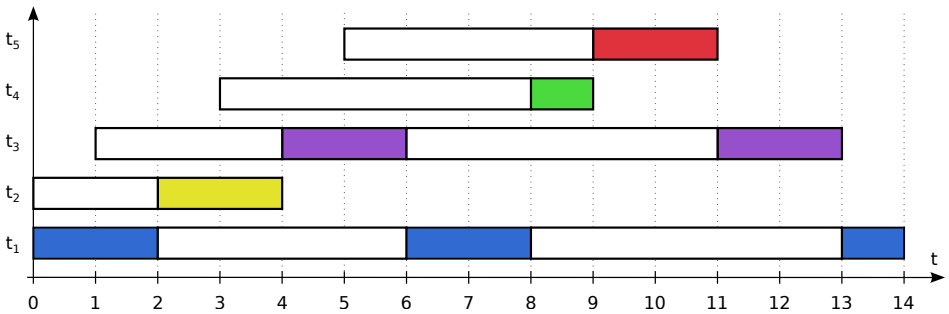
Figura 6.2: Escalonamento Round-Robin .
