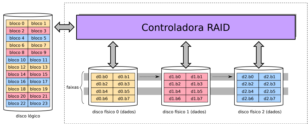
Figura 21.9: RAID nível 0 ( stripping ).
