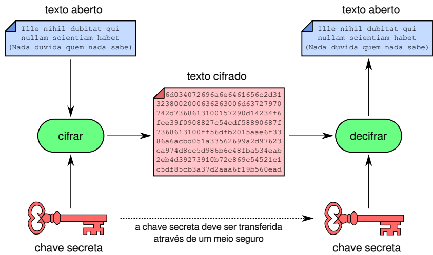
Figura 27.2: Criptografia simétrica.
