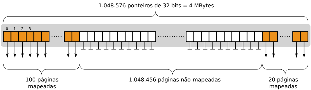
Figura 14.10: Tabela de páginas linear.
