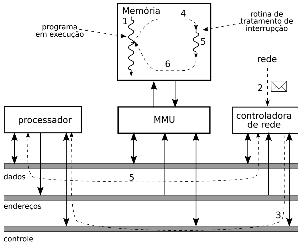
Figura 5: Roteiro típico de um tratamento de interrupção
