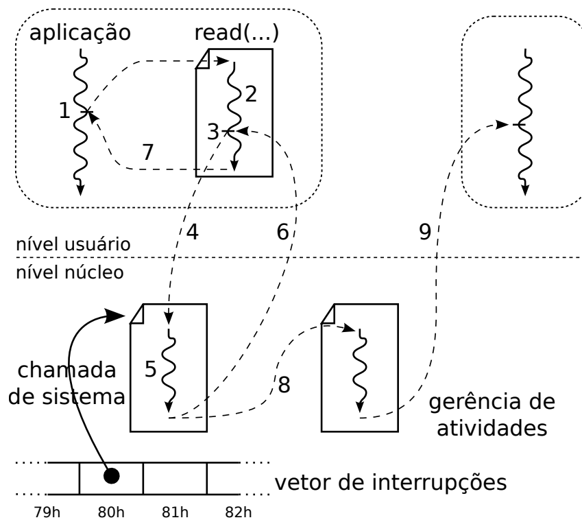
Figura 7: Roteiro típico de uma chamada de sistema
