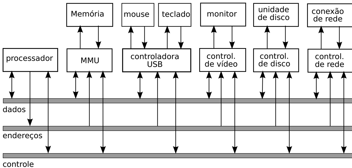
Figura 4: Arquitetura de um computador típico
