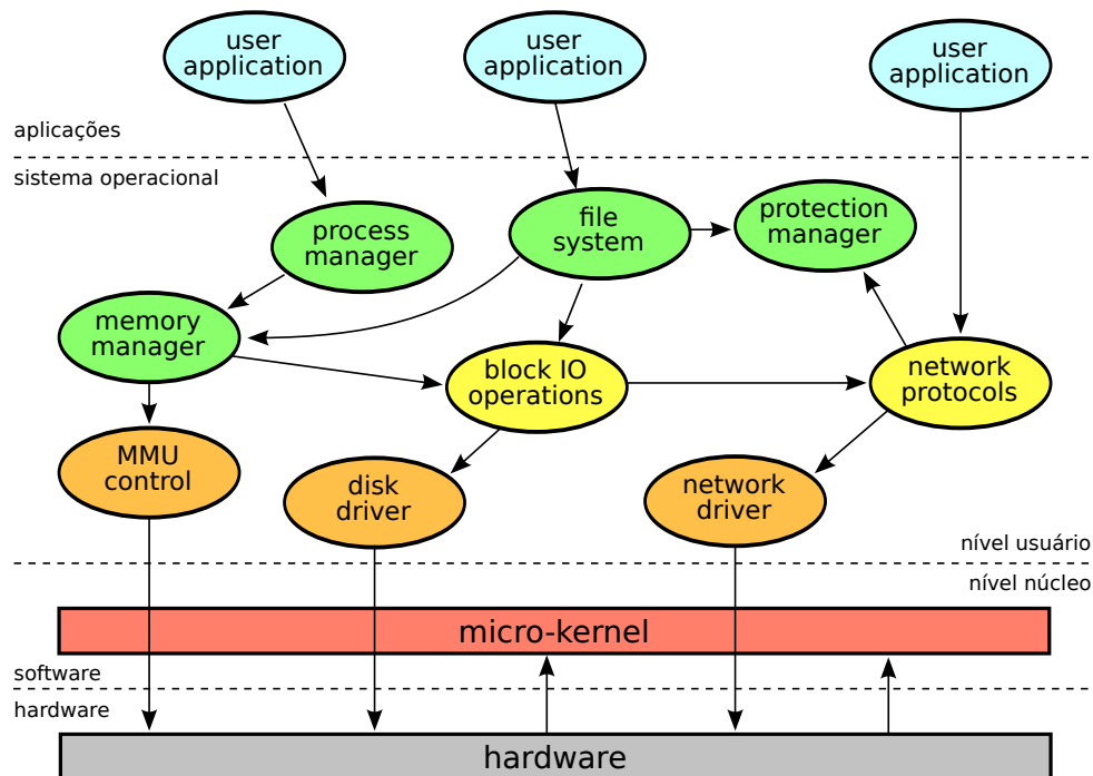
Figura 9: Visão geral de uma arquitetura micronúcleo
