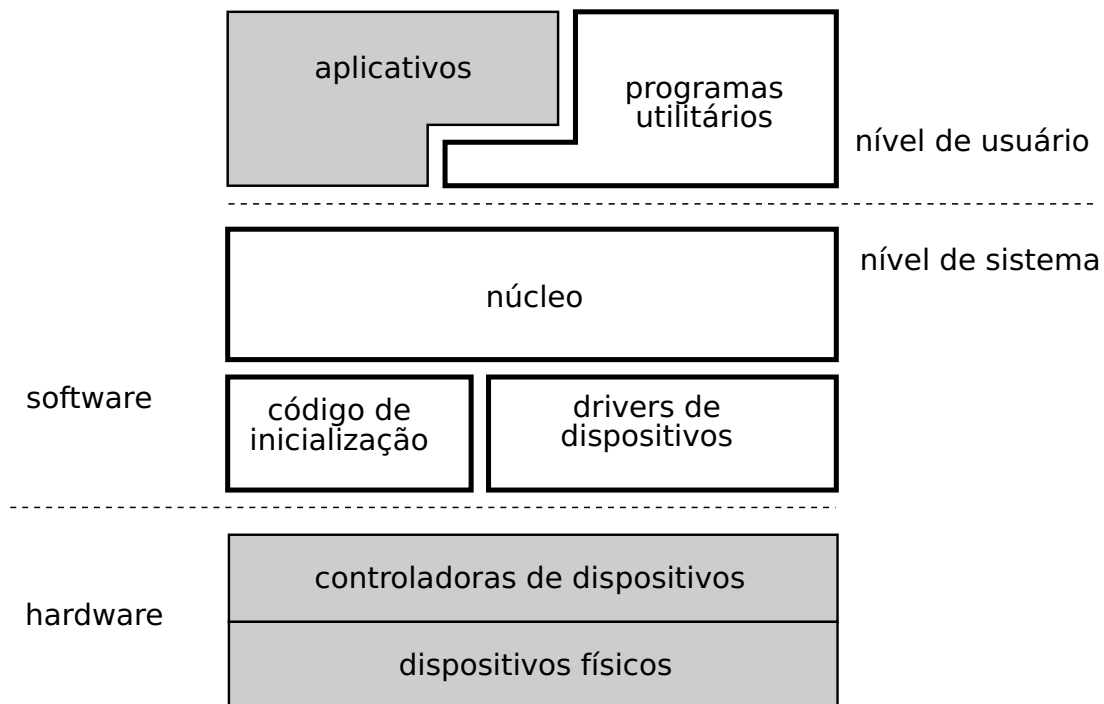
Figura 3: Estrutura de um sistema operacional
