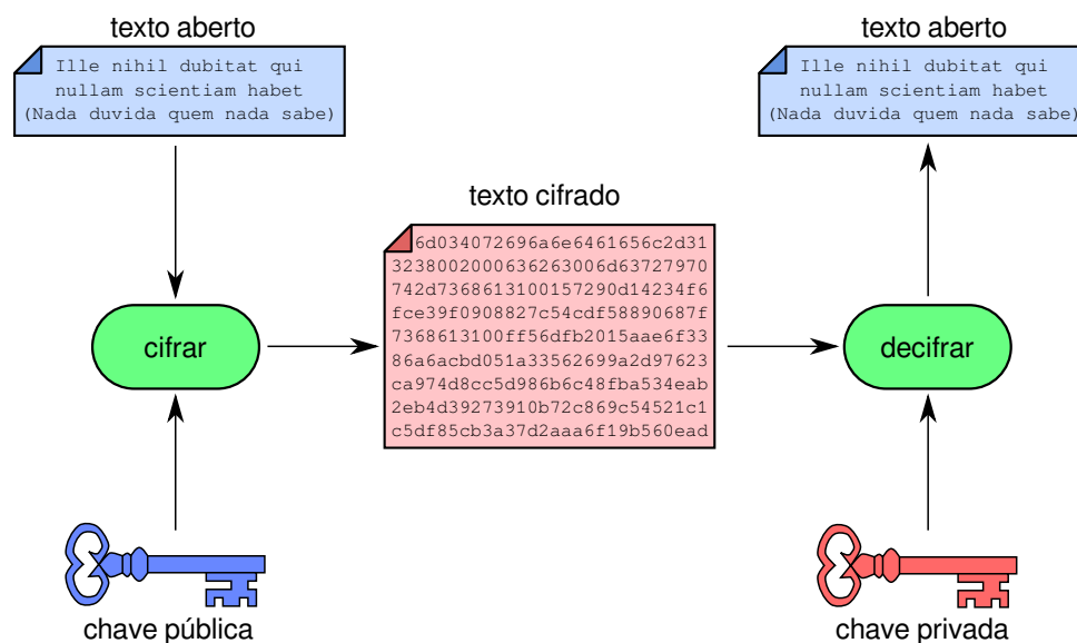
Figura 27.10: Criptografia assimétrica.
