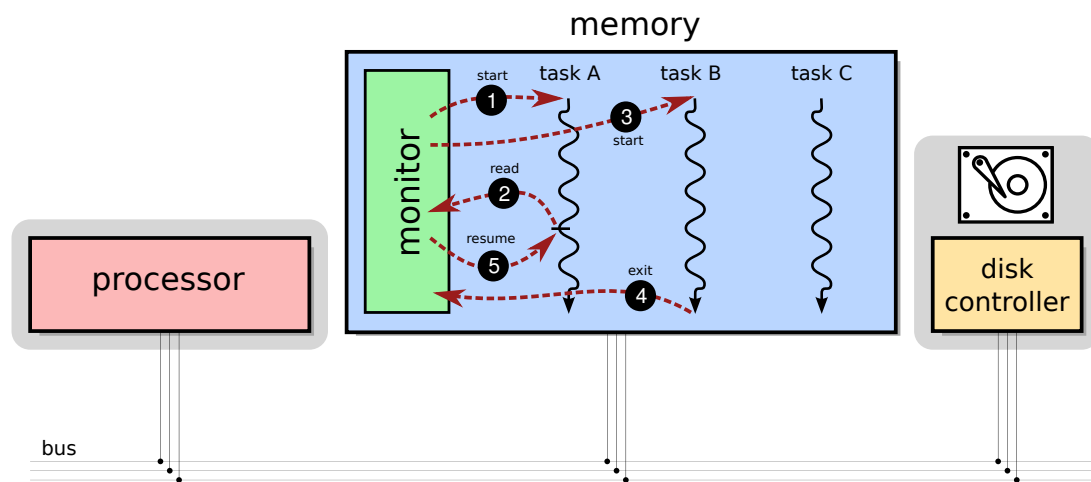
Figura 4.4: Execução de tarefas em um sistema multitarefas.
