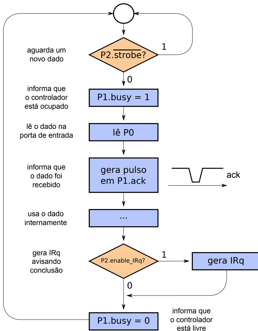
Figura 19.5: Comportamento básico do controlador da porta paralela.
