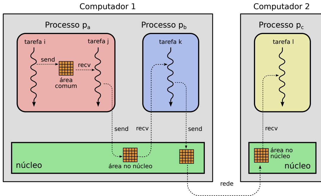
Figura 8.1: Comunicação intraprocesso ( t_i \rightarrow t_j ), interprocessos ( t_j \rightarrow t_k ) e intersistemas ( t_k \rightarrow t_l ).
